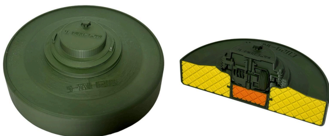
Макет протитранспортної фугасної міни «ТМ-62ПЗ» / «ТМ-62ПЗ» у розрізі
