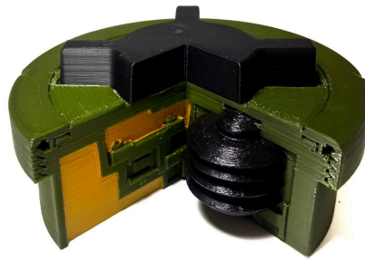
Макет протипіхотної фугасної міни натискної дії «ПМН-2» в розрізі
