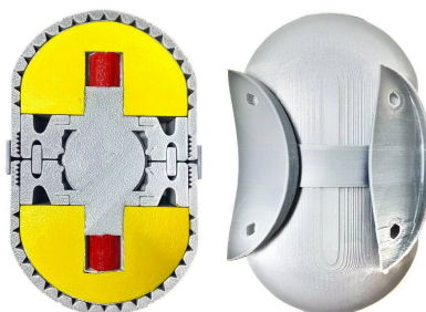
Макет протипіхотного осколково-фугасного суббоєприпасу «АО-2,5 РТ» у розрізі
